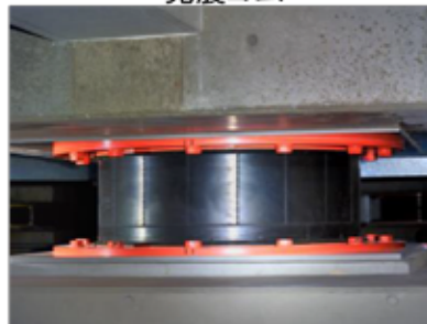
免震ゴム
